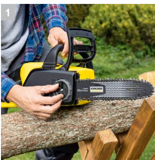
1 Τέντωμα της αλυσίδας χωρίς εργαλεία
